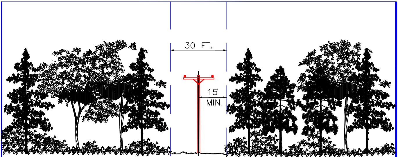
ELEVATION
